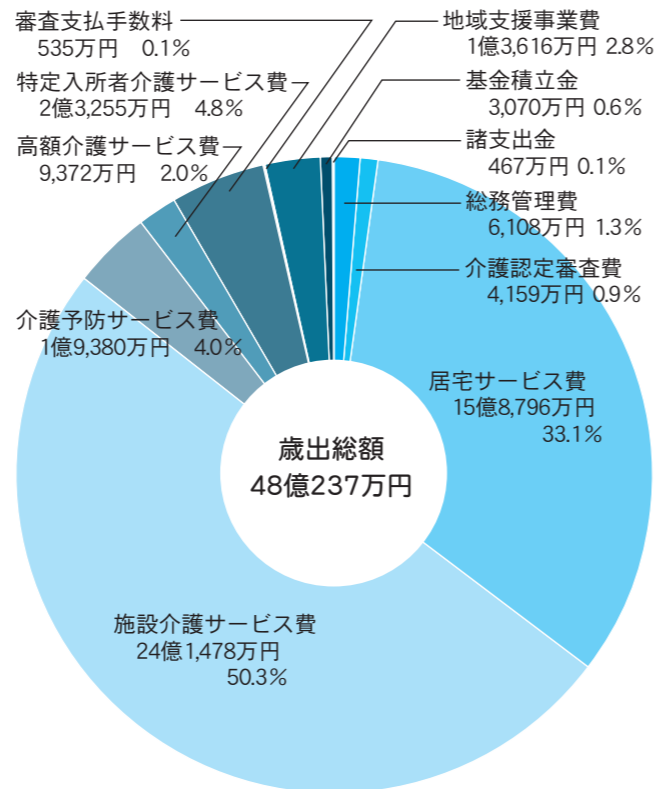
■図2 歳出内訳
