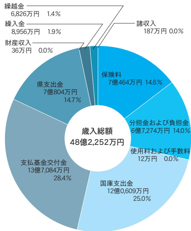
■図1 歳入内訳
